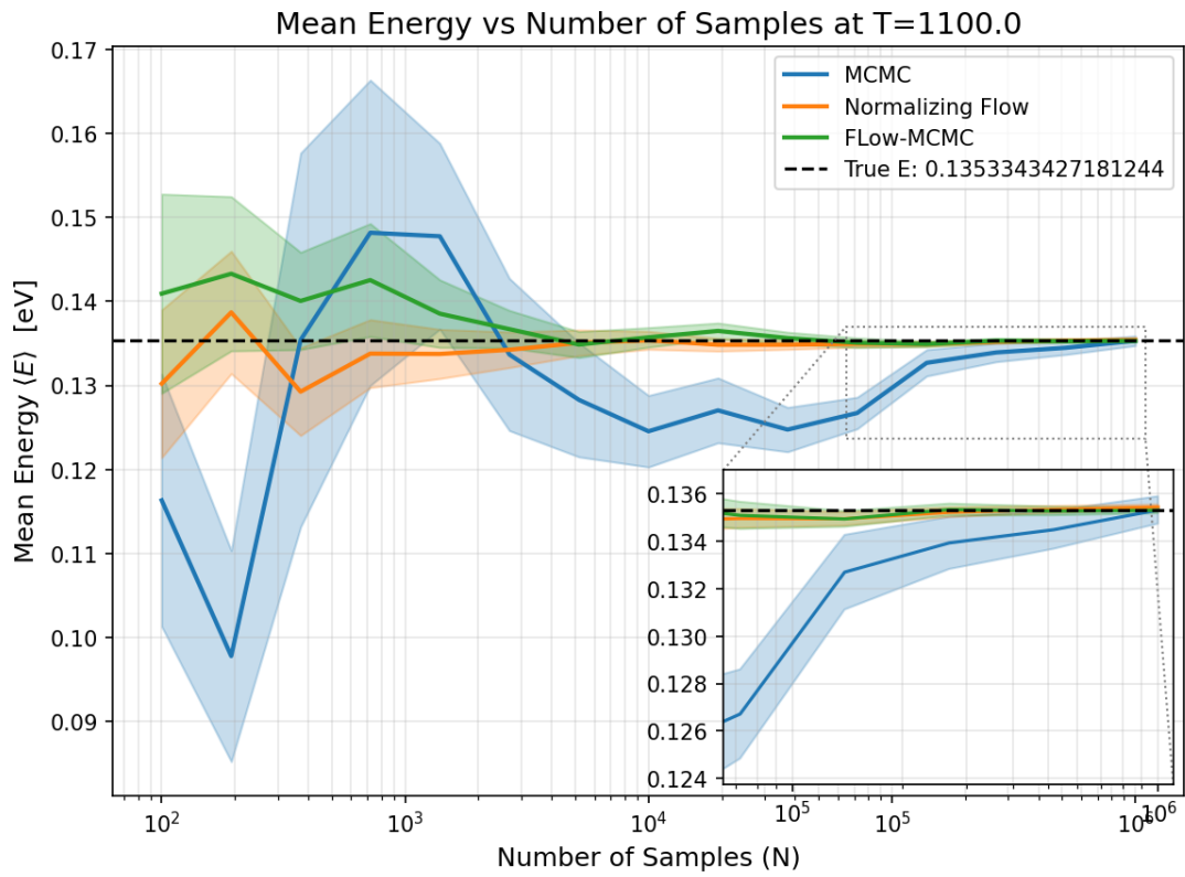
Figura 4.12: Energia media stimata da MCMC, NF e Flow-MCMC in funzione del numero di campioni N , per D = 3 a tre diverse temperature T = 100, 600, 1100 K. La linea tratteggiata indica il valore di riferimento.
